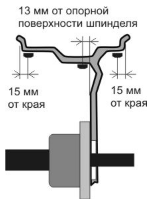
Рисунок 5.16 – Дистанции установки ленточных грузов вручную
