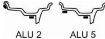
Рисунок 5.6 – Схемы расположения грузов, для которых применяется прямое измерение
